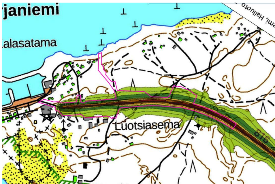
kuva 12. Suunnittelualueen päiväaikainen keskiäänitaso vuonna 2050 tiesuunnitelman mukaisessa tilanteessa.
