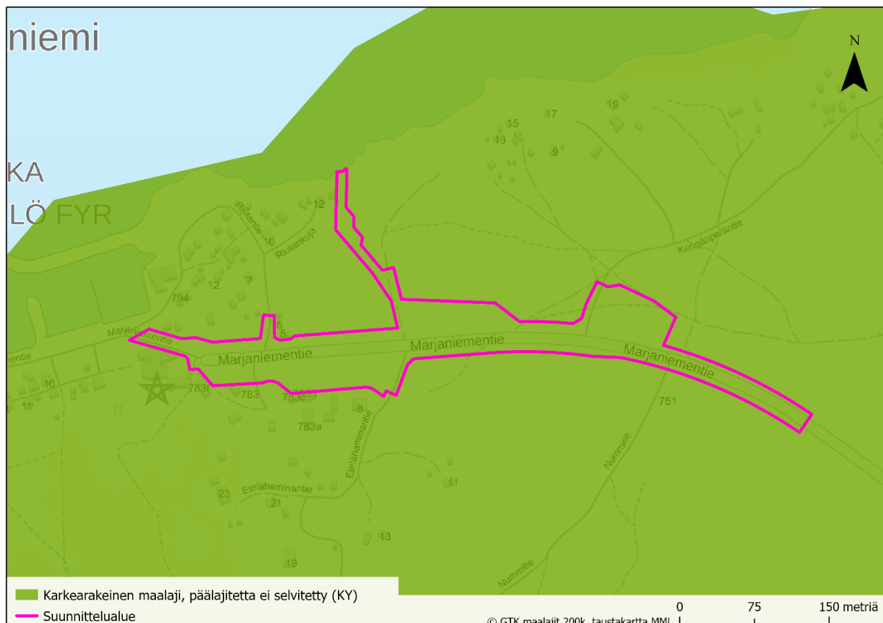
kuva 14. Suunnittelualueen maaperä.
